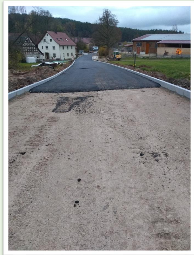
Asphaltierungsarbeiten BT 19 in Prebitz 2021
